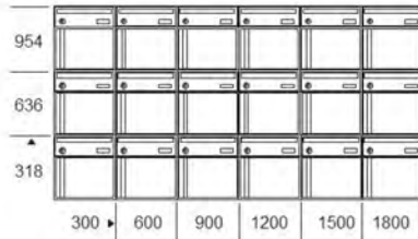
Dimensioni senza rivestimento - Masse ohne Verkleidung - Dimensions sans revêtement
